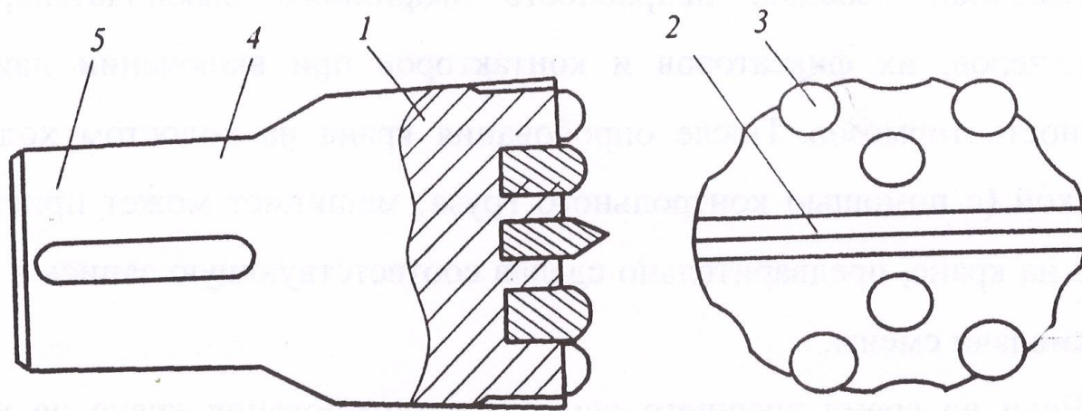
Рис. 1. Схема бурового долота: 1 — головка; 2 — лезвие; 3 — штыри; 4 — корпус; 5 — хвостовик
