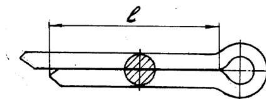
Рис. 1. Шплинт
