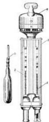
Рис. 3.3 Психрометр Ассмана
