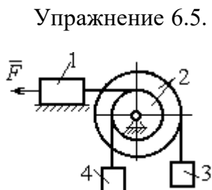
Рис. 6.30. Схема подъёмника
