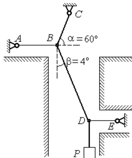
Рис. 1.13. Схема отвеса
