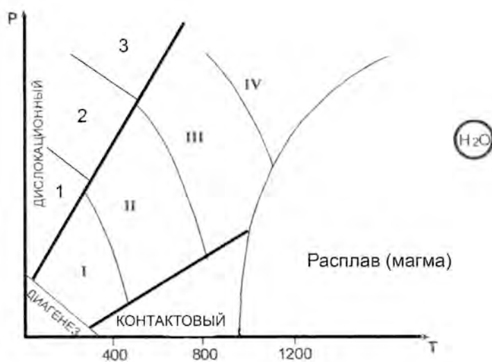
Рис. 1. Типы метаморфизма
