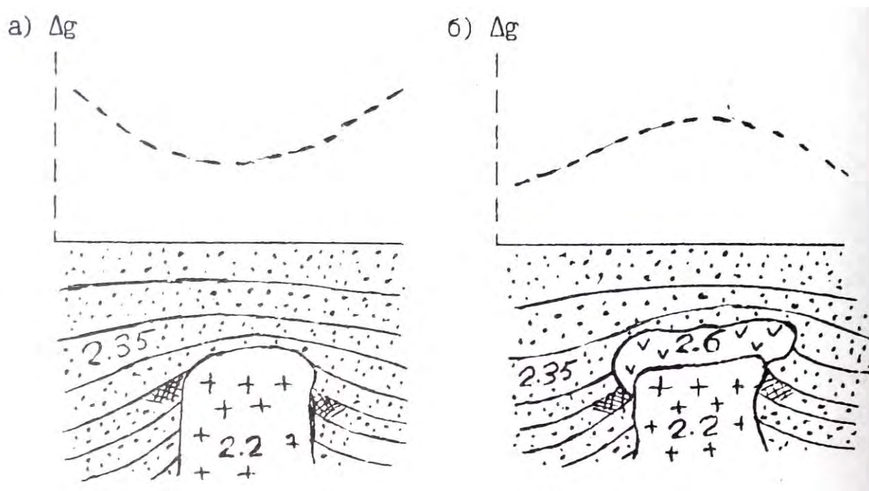
Рис. 3.4. Характер распределения плотности и ускорение силы тяжести над соляно-купольными структурами (×× песчано-глинистые отложения, + - каменная соль, √ — ангидрит, - - - - приращение ускорения силы тяжести, // - нефтеносность)
