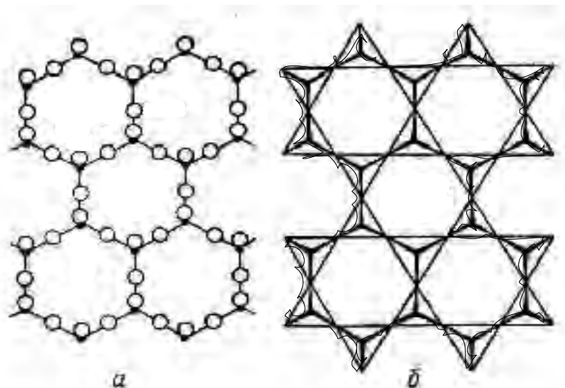
Рис. 5. Кремнекислородный лист [\text{Si}_4\text{O}_{10}]^{4-} : а – разреженная модель; б – в тетраэдрах
