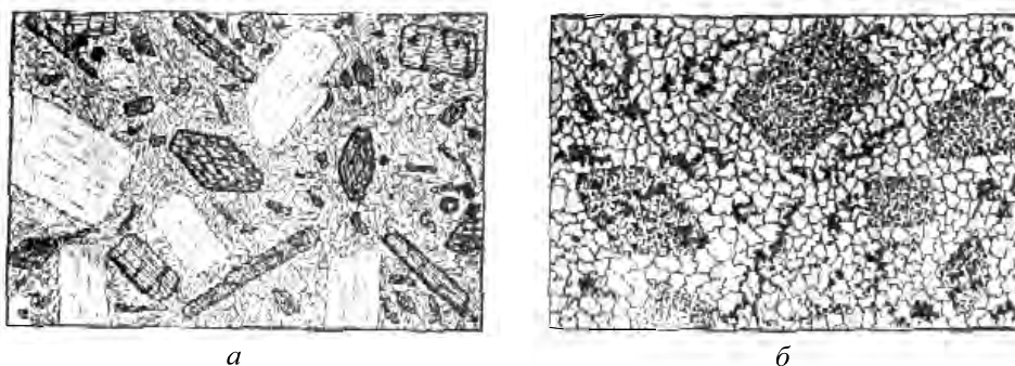
Рис. 27. Березитизация диоритового порфирита (по Б. И. Омеляненко):
