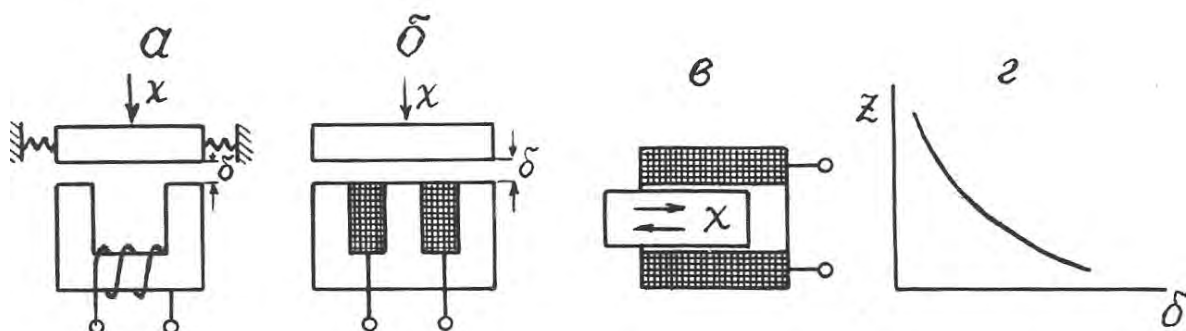
Рис. 2.10. Варианты выполнения индуктивных преобразователей с изменяемым воздушным зазором (а-в) и их статическая характеристика (z).
