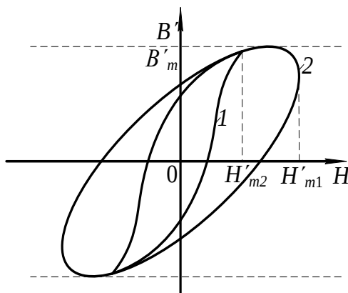
Рис. 3.26. Свойство динамических петель намагничивания с постоянной магнитной индукцией и различной частотой магнитного поля
