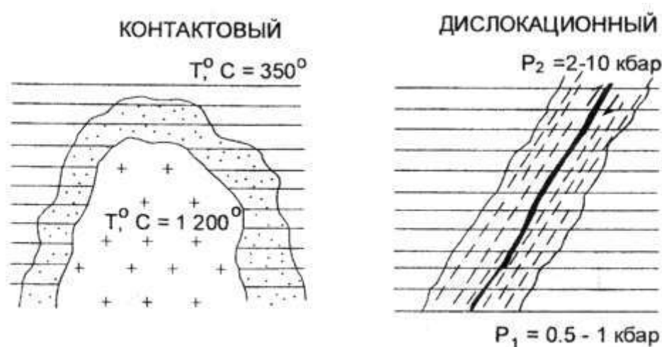
Рис. 3. Локальные типы метаморфизма
