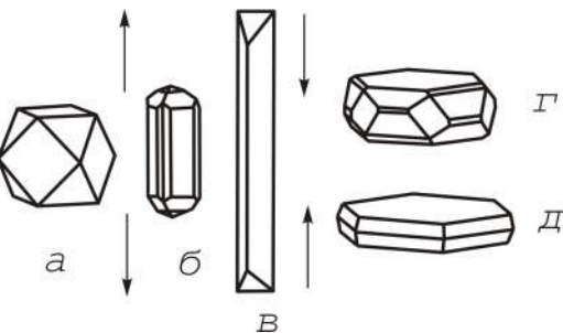
Рис. 3. Типы облика кристаллов: а – изометричный; б – короткопризматический; в – длиннопризматический; г – таблитчатый; д – пластинчатый.
