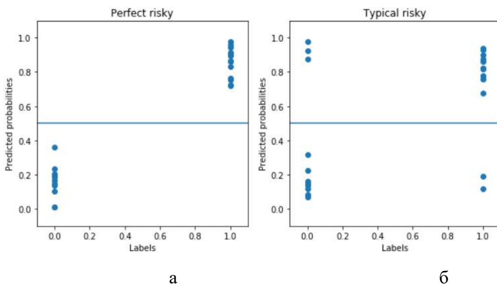
Рисунок 4 – Примеры действительного и предсказанного векторов для идеального (а) и типичного (б) рисковющего алгоритма
