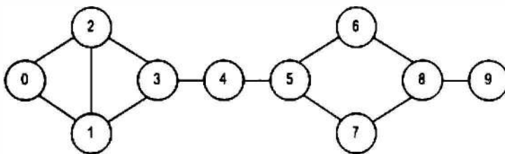
Рис. 1.1. Сеть DataSciencecenter
