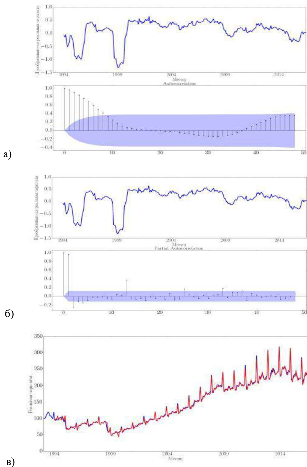
Рисунок 38 – (а) Коррелограмма со значениями автокорреляций временного ряда с удалённым трендом; (б) график частичных автокорреляций временного ряда; (в) исходный временной ряд (синяя кривая) и предсказания модели ARMA (2,2) (красная кривая) [3]
