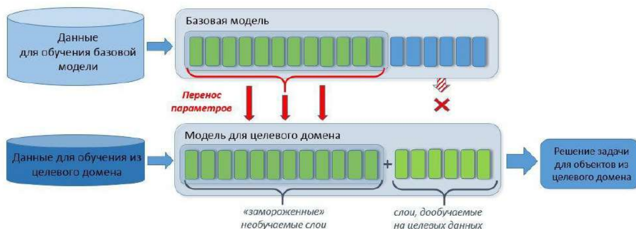
Рисунок 35 – Схема переноса обучения.
