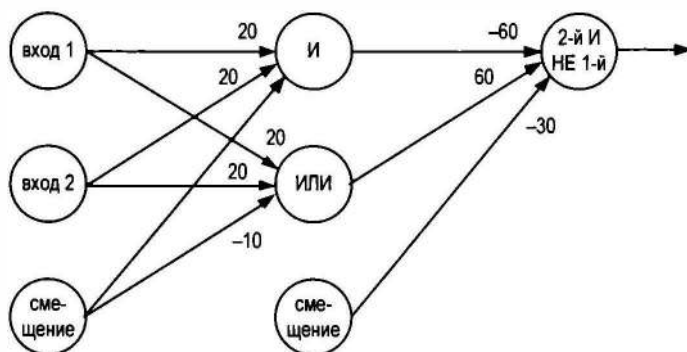
Рис. 18.3. Нейронная сеть для логического вентилля "исключающее ИЛИ"
