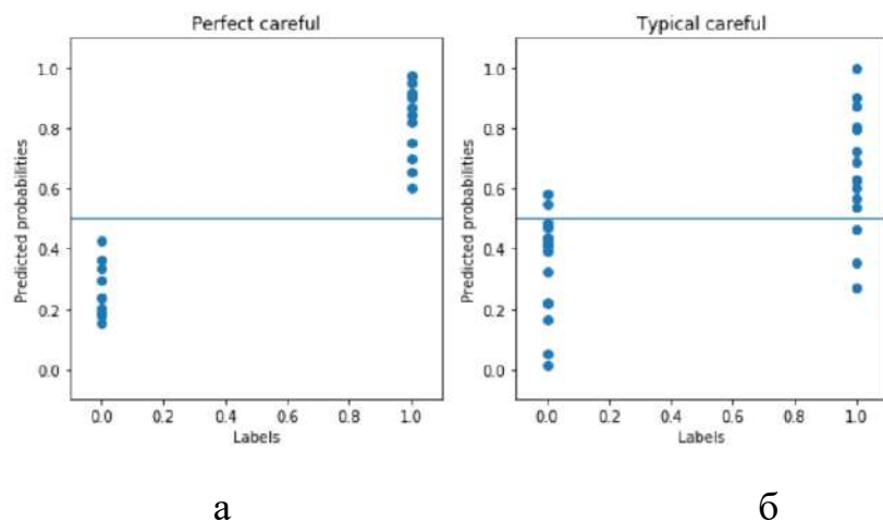
Рисунок 3 – Примеры действительного и предсказанного векторов для идеального (а) и типичного (б) осторожного алгоритма
