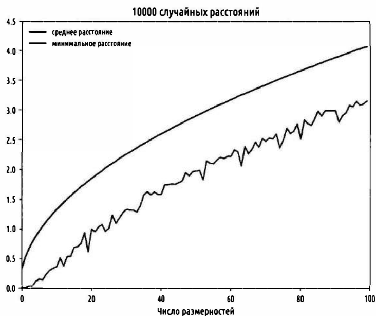
Рис. 12.2. Проклятие размерности
