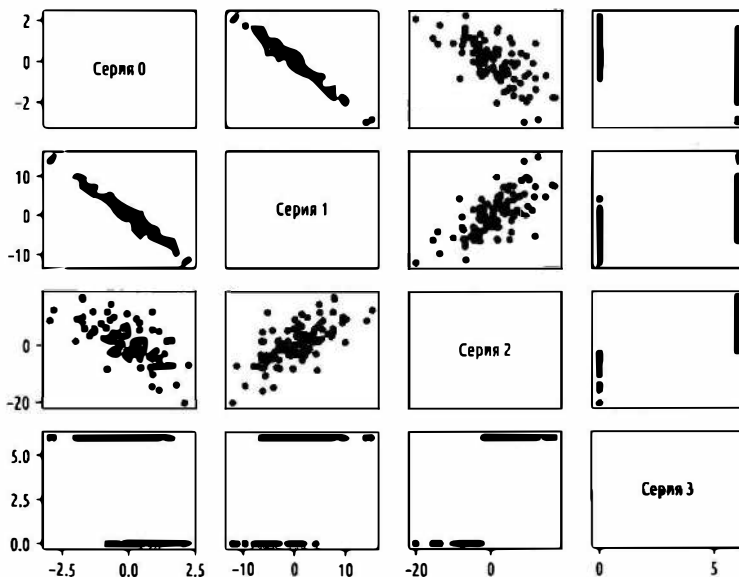
Рис. 10.4. Матрица рассеяний
