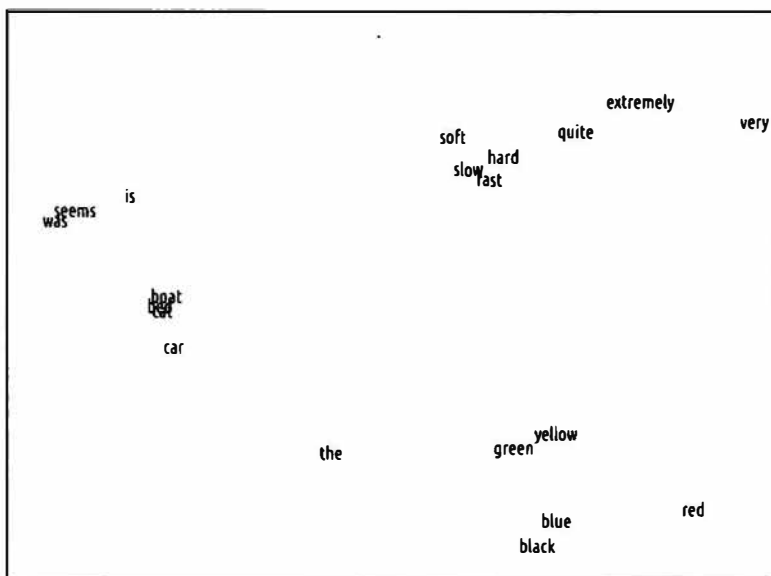
Рис. 21.3. Векторы слов
