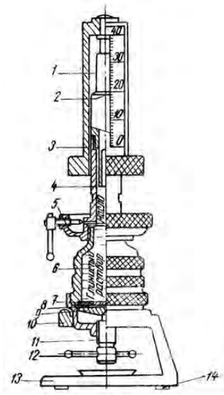
Рис. 3. Прибор ВМ-6 в сборе
