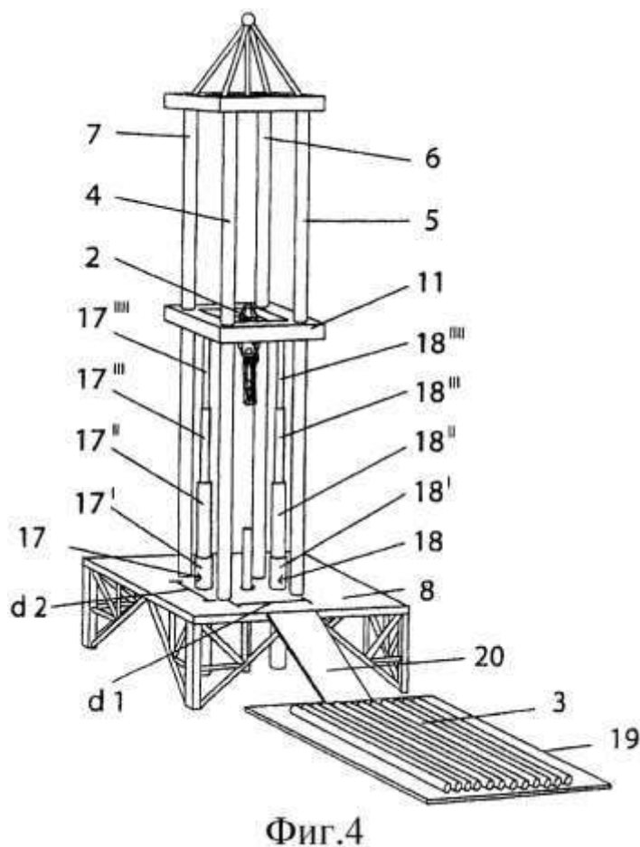
Рисунок 2 – Буровая установка,..... 1
