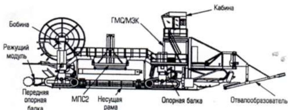
Рисунок 2 – Конструктивная схема комплекса глубокой разработки угольного пласта,..... 1
