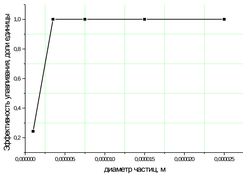
Зависимость эффективности улавливания от диаметра частиц пыли
