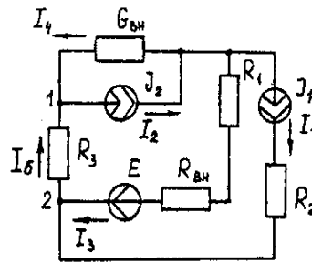
Рис. 1.2. Схема заданной электрической цепи
