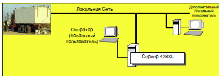
Рисунок 2 – Топология локального пользователя сейсмостанции 428XL 2
