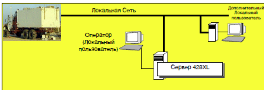
Рисунок 2 – Топология локального пользователя сейсмостанции 428XL 6
