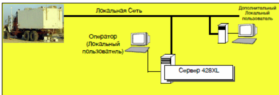
Рисунок 2 – 1 топология локального пользователя сейсмостанции 428XL 4
