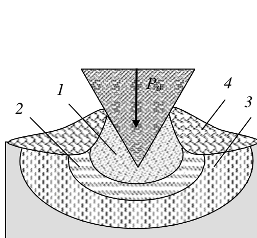
Рис. 1.76. Схема внедрения бурового инструмента в породу: 1 – зона дробления; 2 – зона разрушения; 3 – зона трещинообразования; 4 – зона скола.
