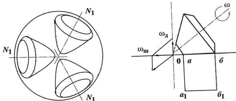
Рис. 2.95. Кинематика одноконусной шарошки: \omega_d - угловая скорость вращения долота; \omega_{ш} - угловая скорость шарошки; \alpha, \alpha_1, \beta, \beta_1 - проекция образующей корпуса шарошки на забой.
