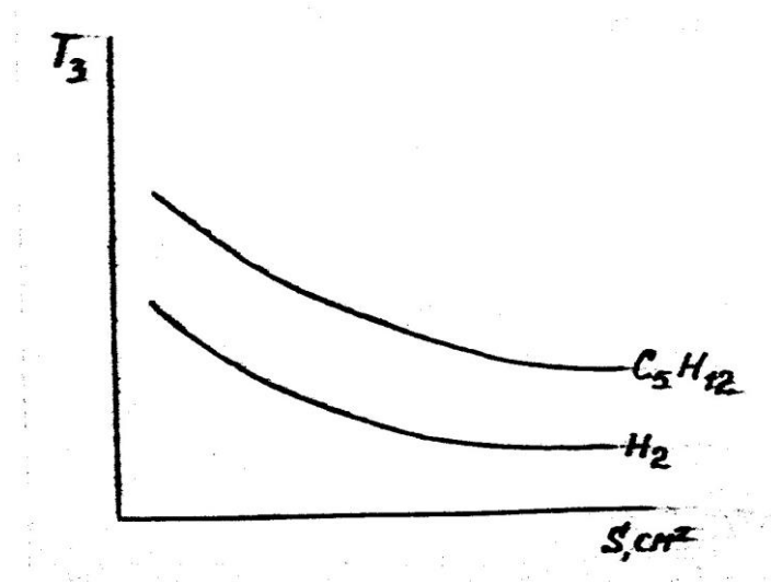
Рис.4. Зависимость критической температуры зажигания от площади поверхности металлического шарика
