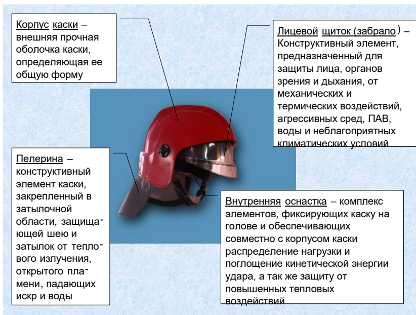
Рис.52 Каска пожарного
