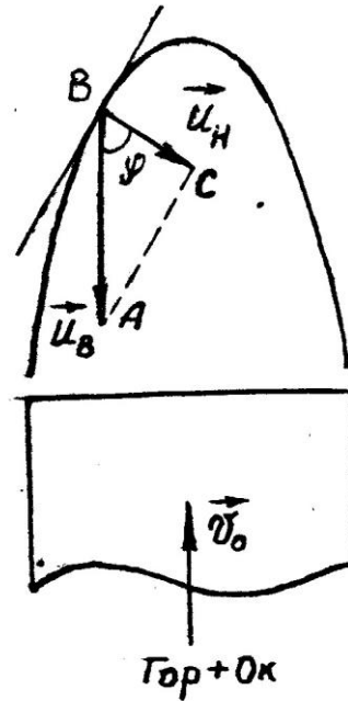
Рис..2. Схема распространения пламени в горелке Бунзена
