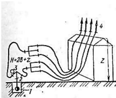
Схема испытания сети свободным изливом воды из пожарных колонок
