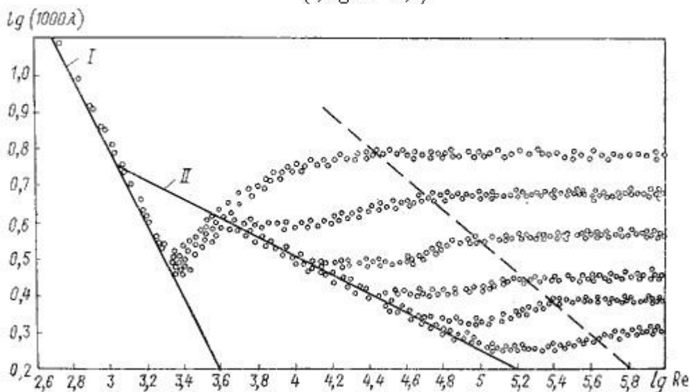
Рис. 4.7. График Никурадзе
