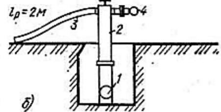
Измерение напора у пожарного крана
