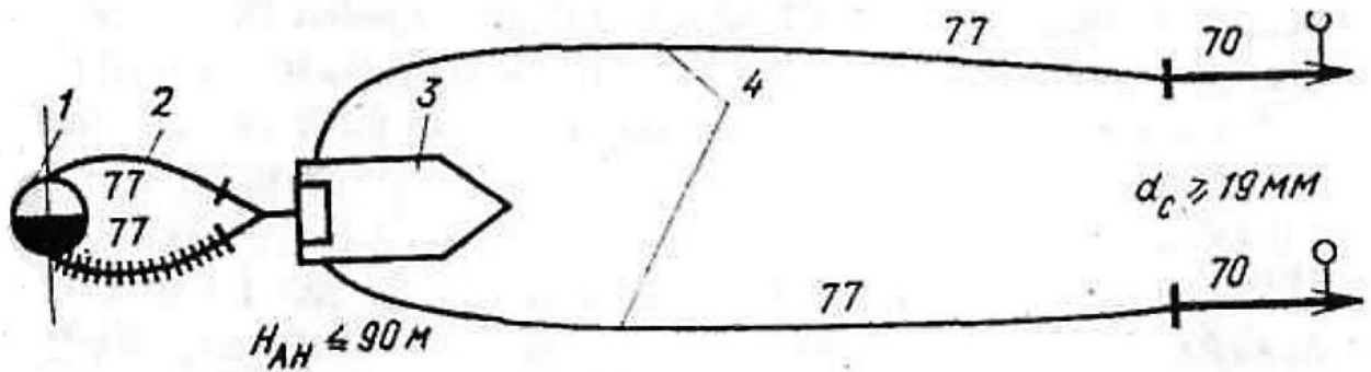
Схема испытания сети отбором воды пожарными автонасосами
