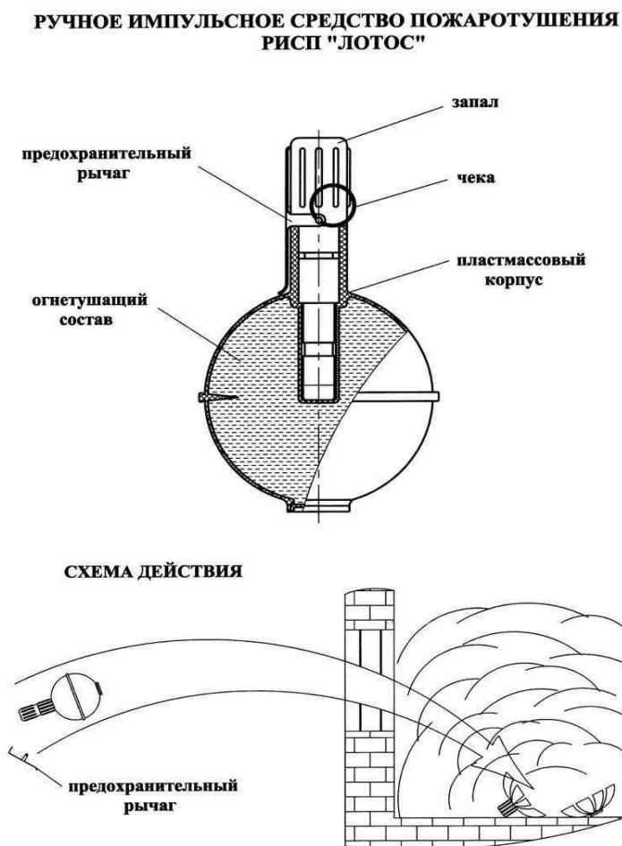
Рис.23. Забрасываемый порошковый огнетушитель РИСП «Лотос» Д-2 Газовые
