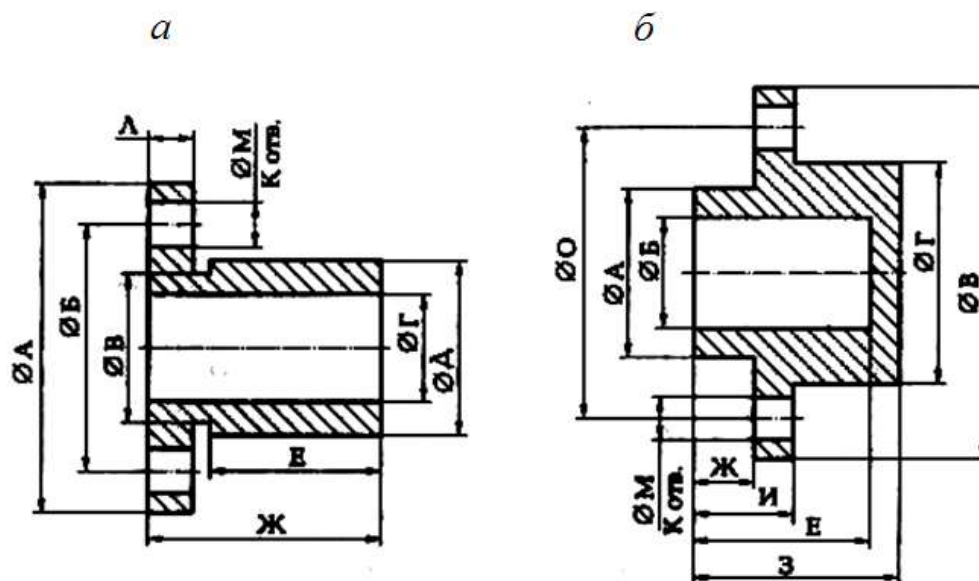
Рис. 1.1. Исходная информация для выполнения контрольной работы : а – первая деталь; б – вторая деталь
