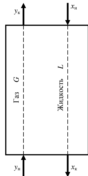
Рис.1. Схема материального баланса
