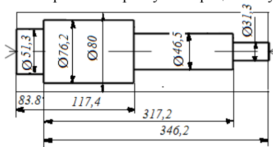
Рис.9 Эскиз детали
