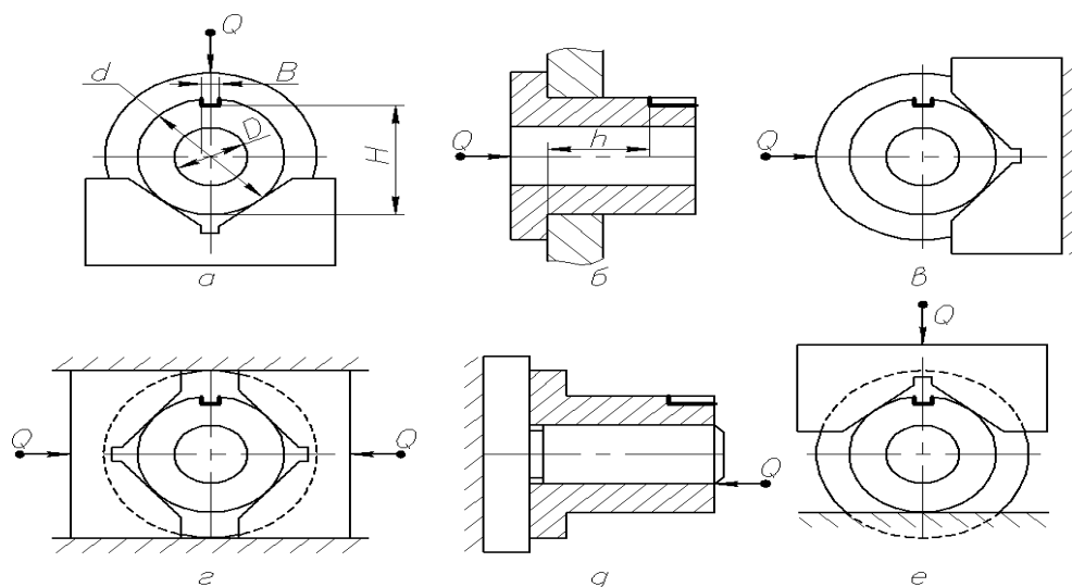
Рис.6 Схемы установки
