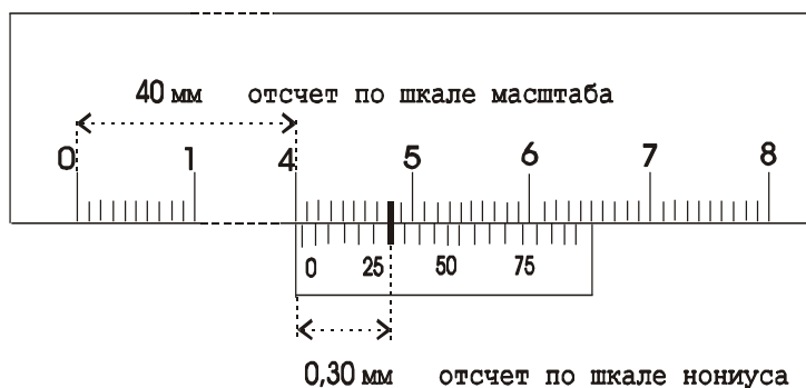
Рис.1.1. Штангенциркуль
