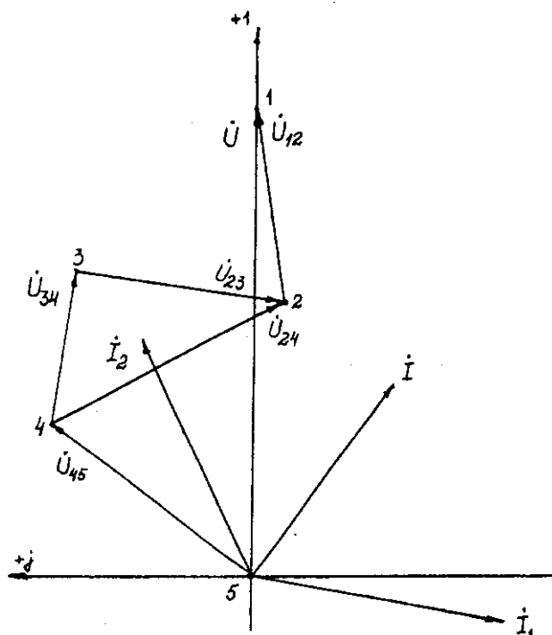
Рис. 2.4. Векторная диаграмма токов и напряжений
