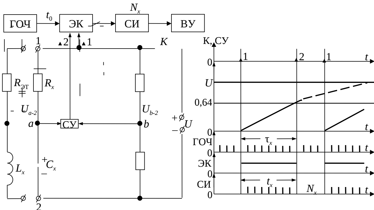
Рис. 2.2. Функциональная схема и временные диаграммы прибора для измерения R, L и C
