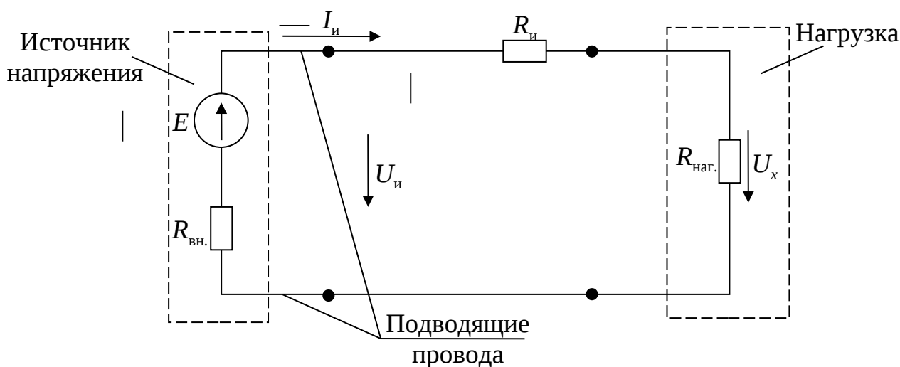
Рис. 1.1. Схема определения значения напряжения расчетным путем
