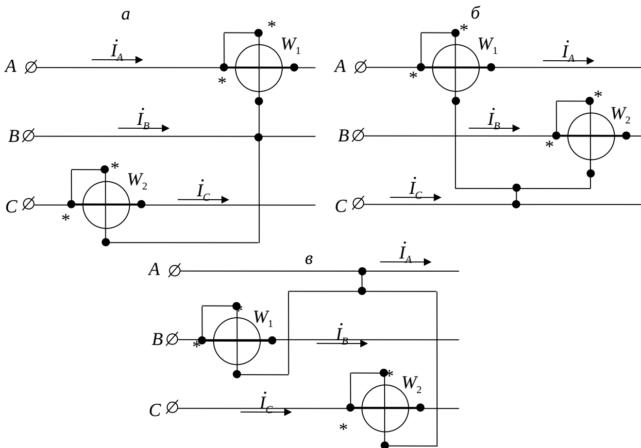
Рис. 3.6. Схемы включения двух однофазных ваттметров для измерения активной мощности 3-фазной 3-проводной цепи а – схема включения фаз A-C; б – схема включения фаз A-B; в – схема включения фаз B-C
