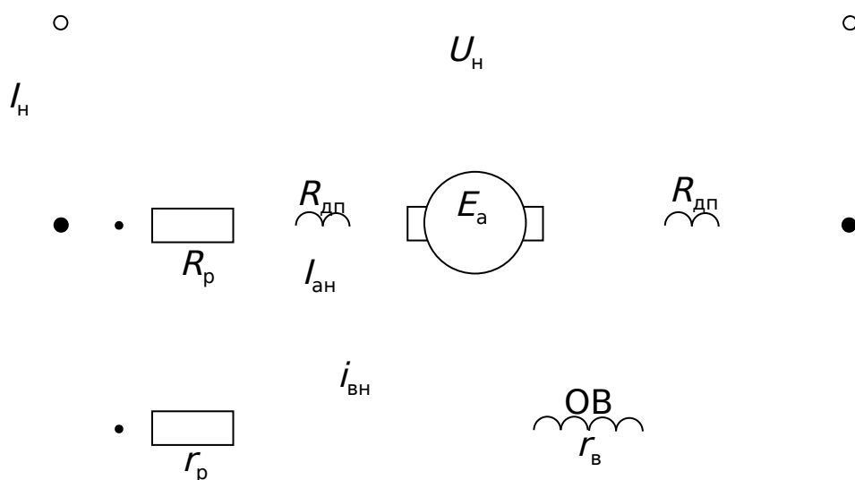
Рис. 6.1. Поясняющая электрическая схема для решения расчетно-графической работы
