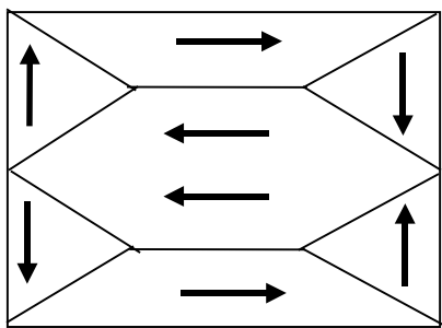
Рис. 1. Доменная структура ферромагнетика
